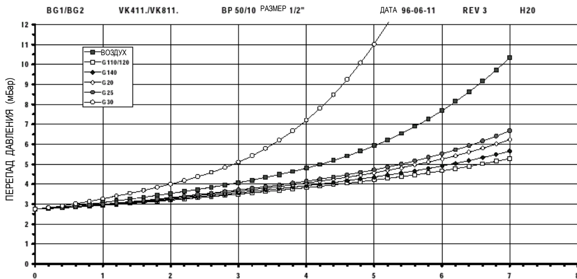
РАСХОД (м³/час) при сухом воздухе, давлении 1013 мБар и температуре 15°C
