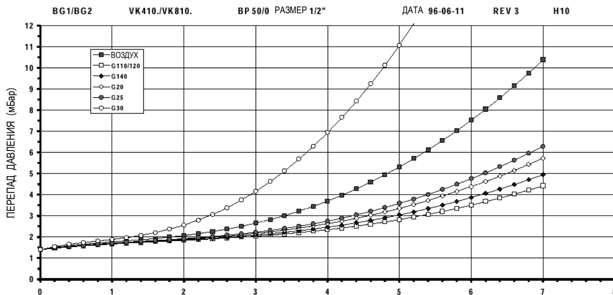
РАСХОД (м³/час) при сухом воздухе, давлении 1013 мБар и температуре 15°C
